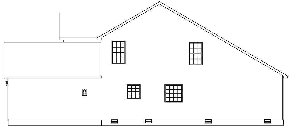
RIGHT ELEVATION
