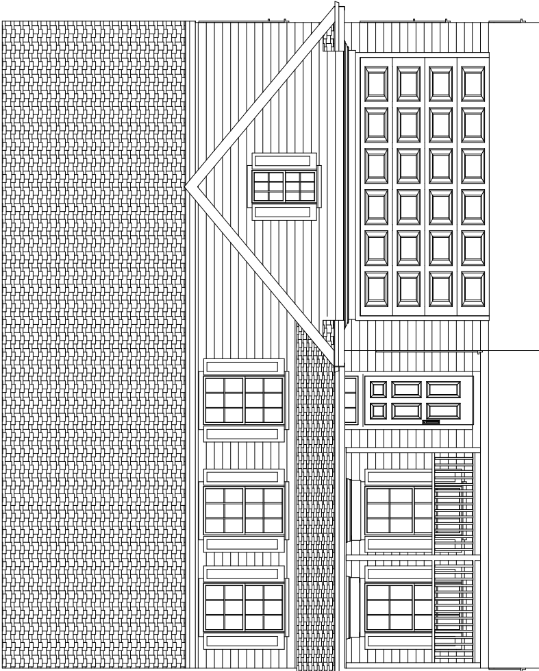
ELEVATION 2
