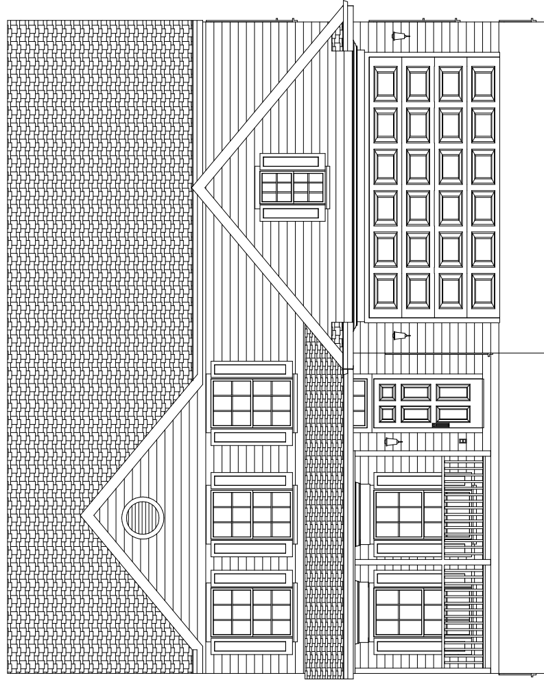
ELEVATION 3
